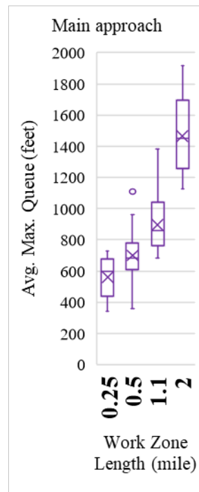
d. Queue for V_{Comb} of 150_100
