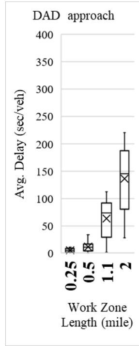
a. Delay for V_{Comb} of 50_25
